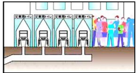
マンホールトイレの事例図
